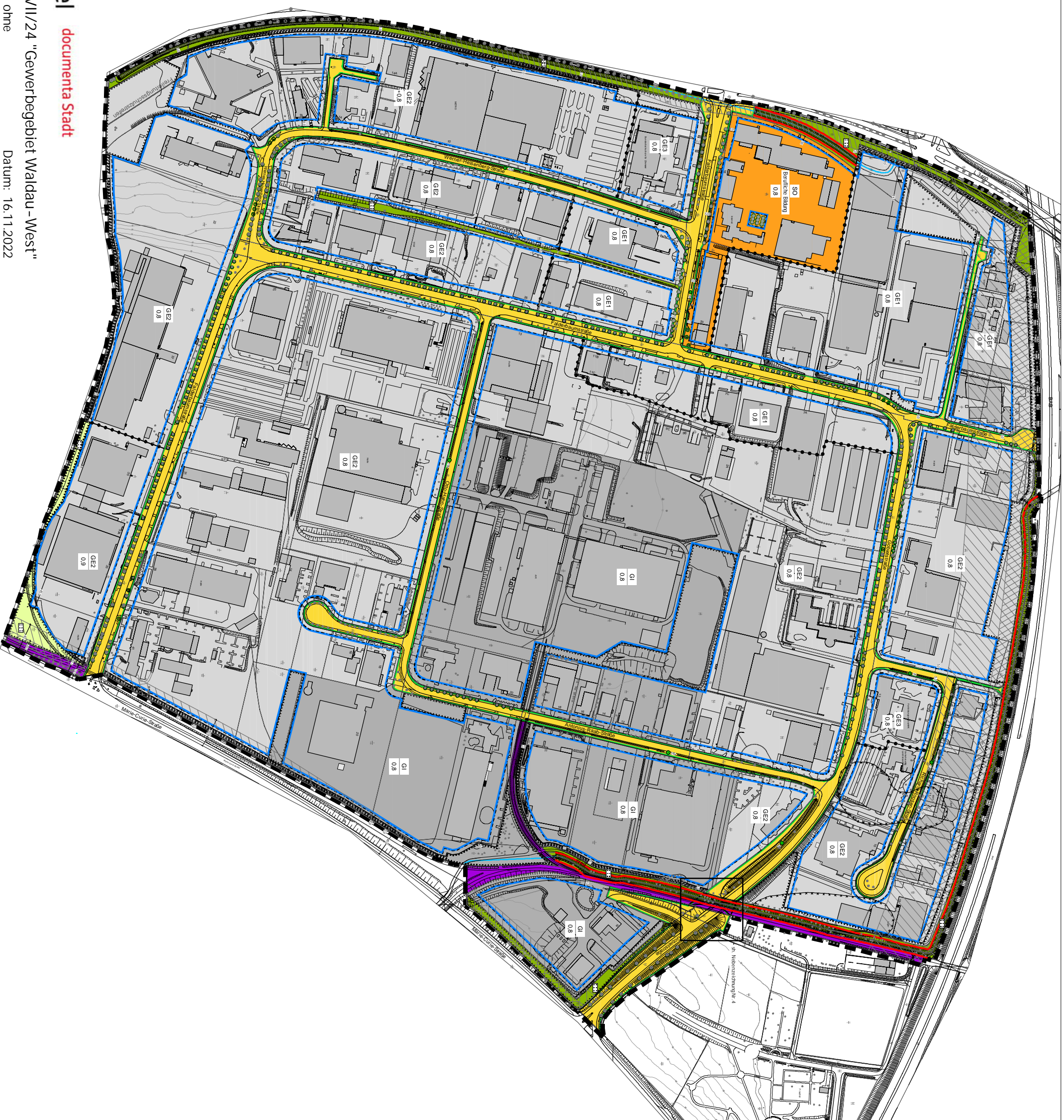
Nebenzeichnung 1: Gliederung des Plangebietes bzgl. Störfallanlagen nach KAS -18 sowie auszuschießenden Abstandsklassen gem. Abstandsklass NRW sh. textliche Festsetzungen 1.2.1 und 1.2.2
